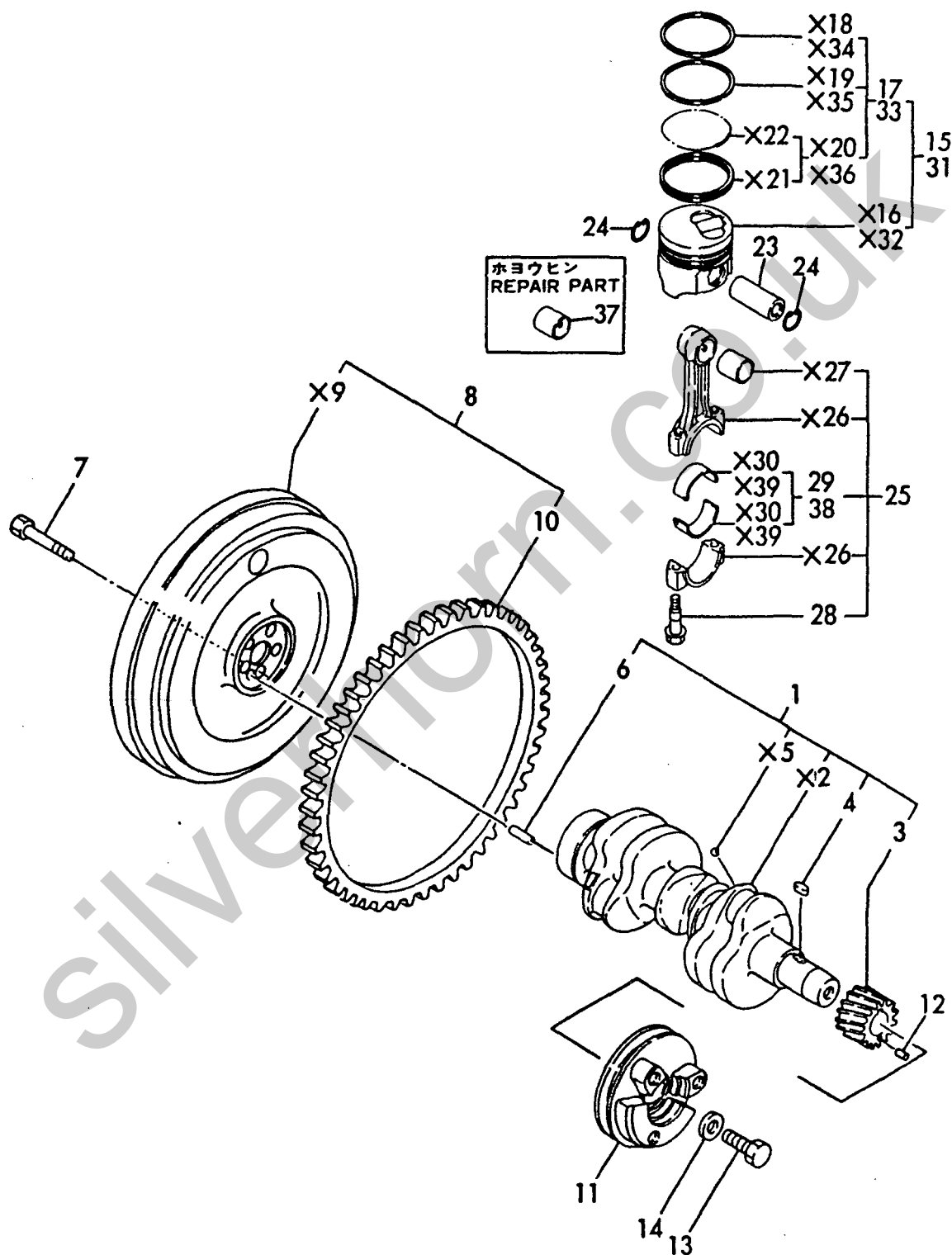
Fig. 7 クランクシャフト & ピストン CRANKSHAFT & PISTON
