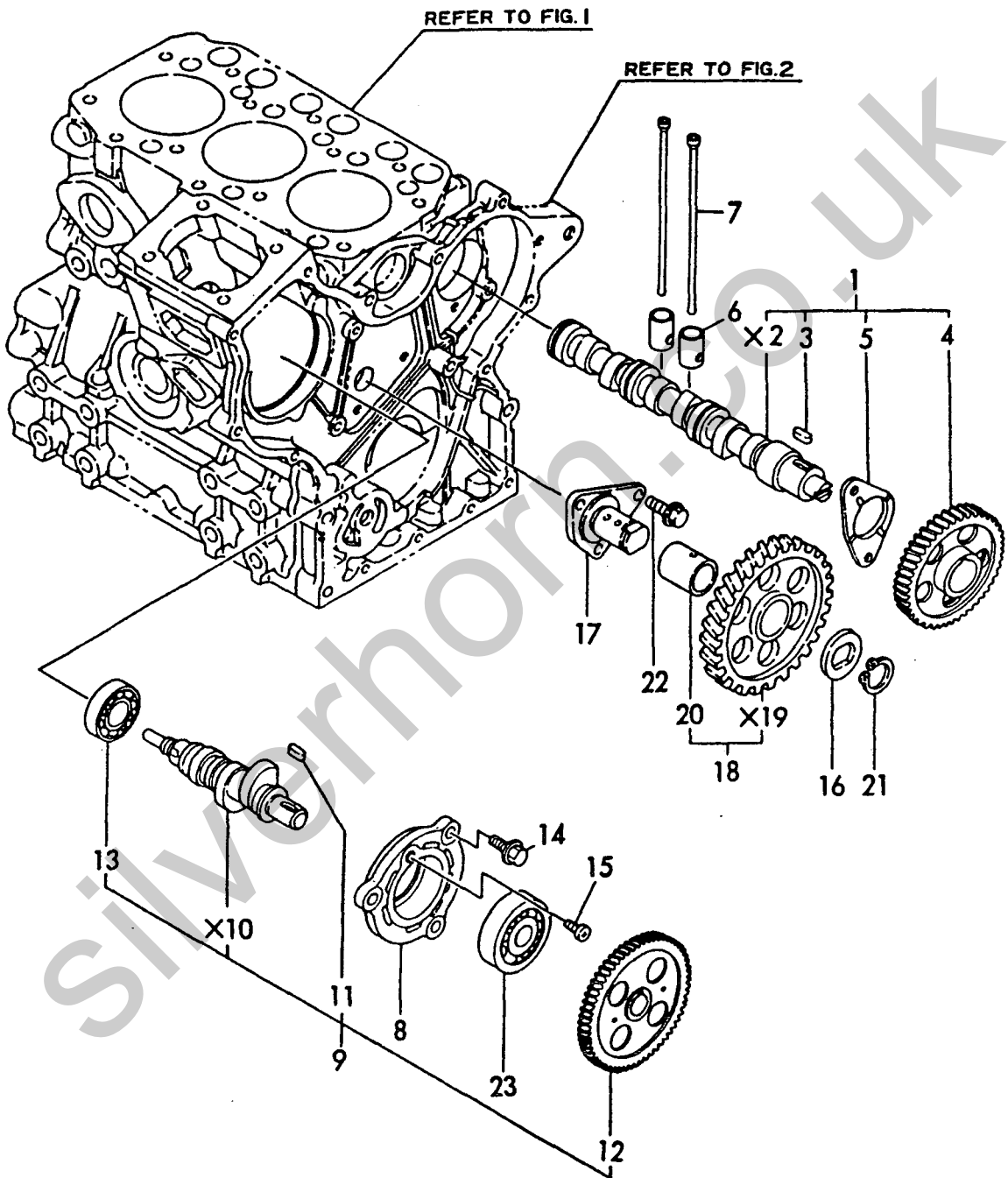
Fig. 6 カムシャフト&クドウギヤ CAMSHAFT & DRIVING GEAR
