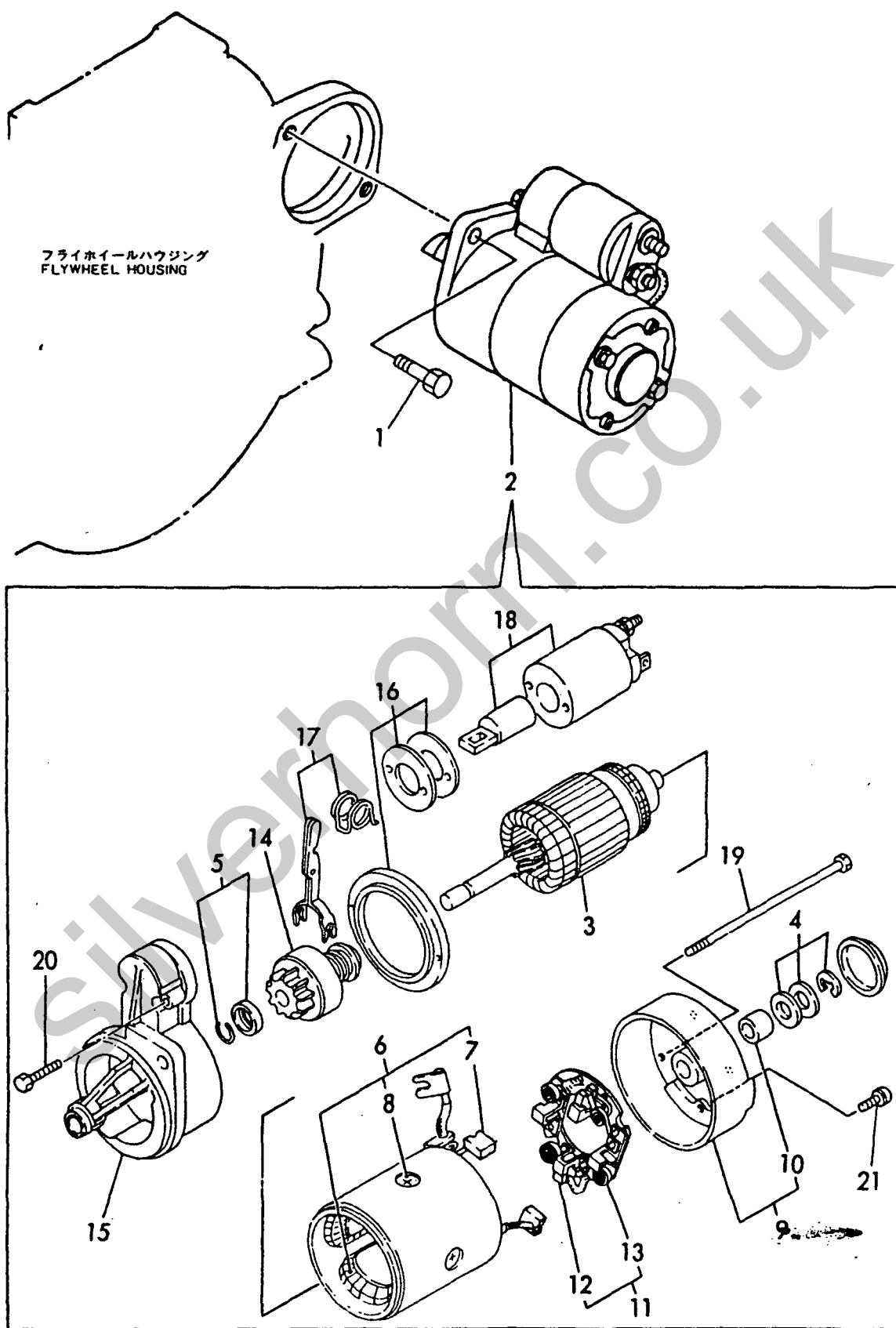
Fig. 13 スターティングモータ STARTING MOTOR
