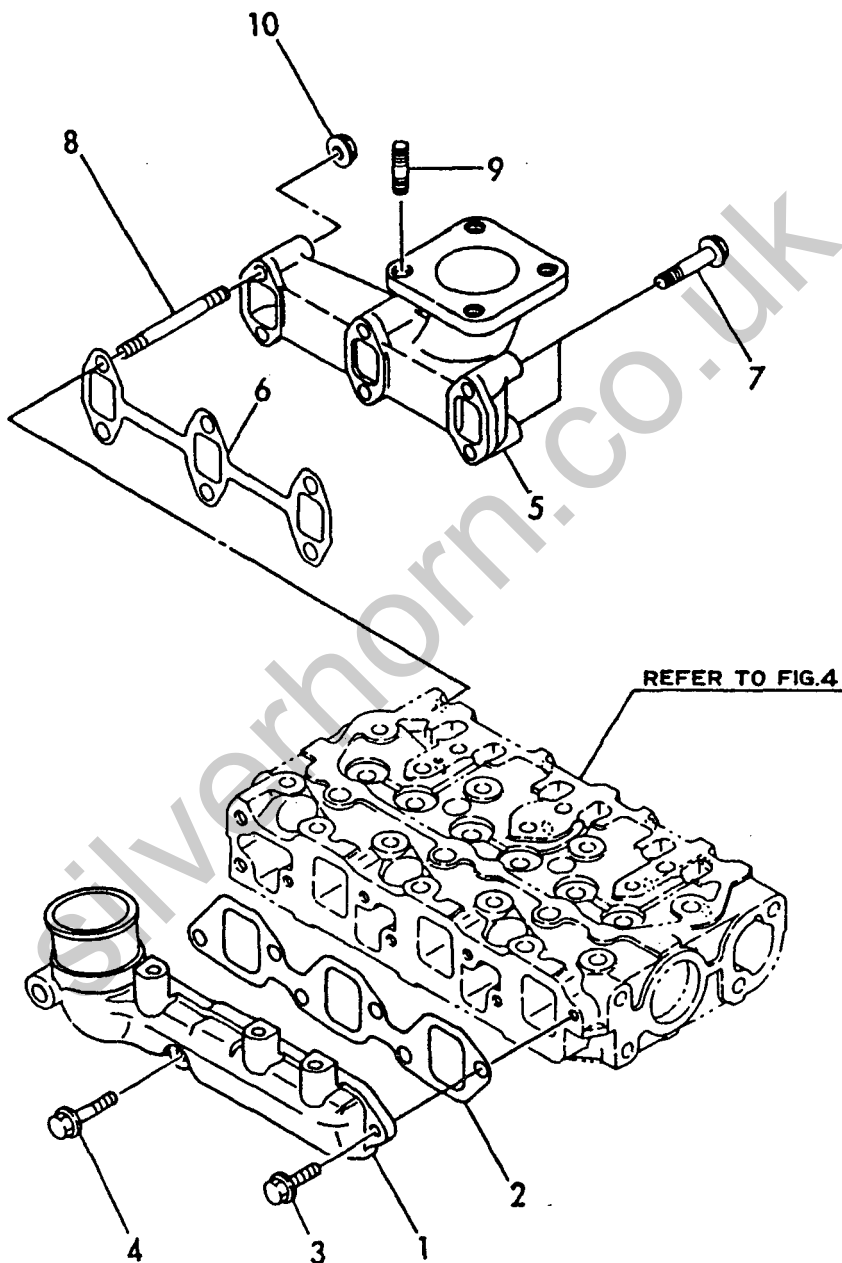
Fig. 5 キュウキマニホールド&エアクリーナ SUCTION MANIFOLD & AIR CLEANER
