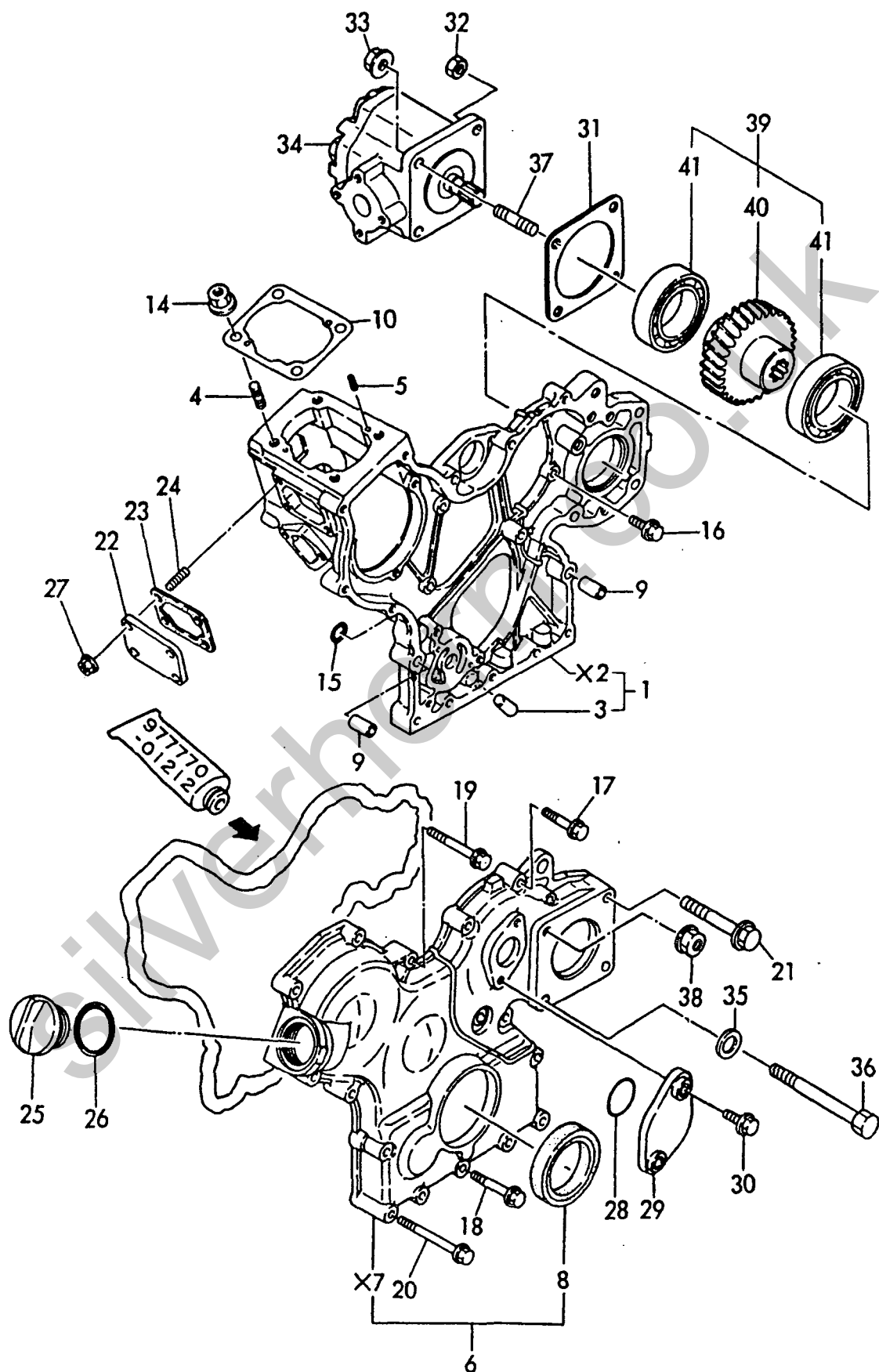
Fig. 2 ギヤケース GEAR HOUSING
