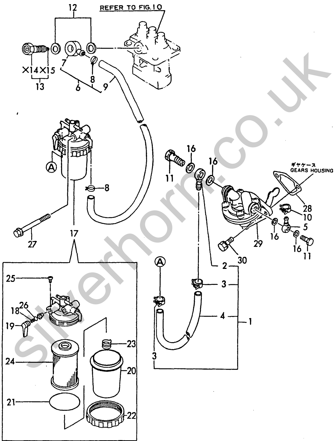
Fig. 11 FOパイプ FUEL LINE
