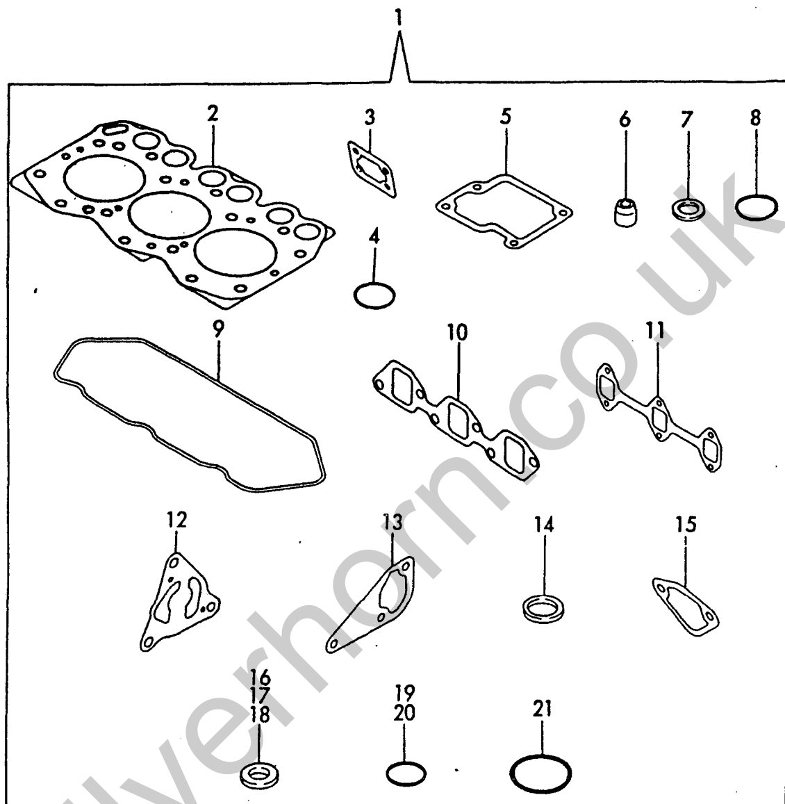
Fig. 15 パッキンセット&コウグ(オプション) GASKET SET & TOOL (OPTIONAL)
