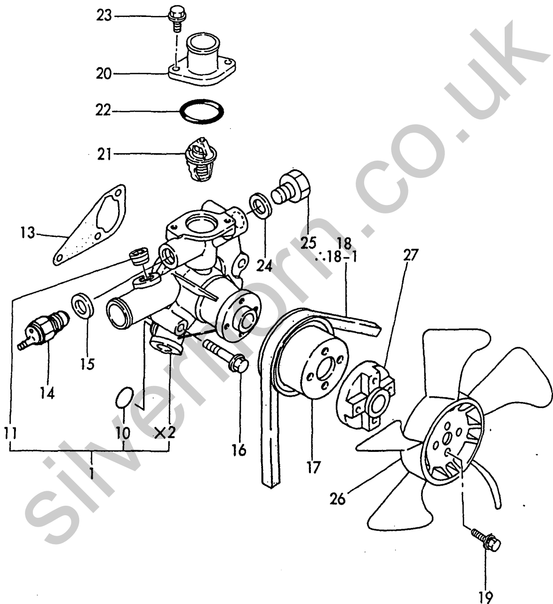
Fig. 9 CWシステム COOLING WATER SYSTEM
